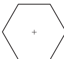
hexagone régulier
