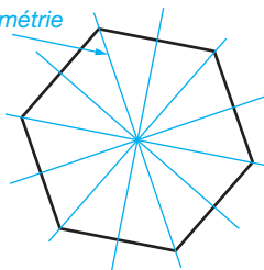
hexagone régulier
