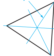
triangle équilatéral
